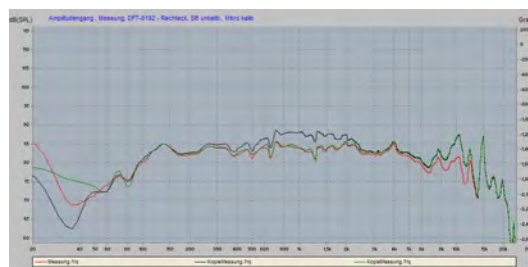
Amplitudengang 10° seitlich
