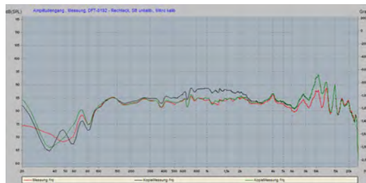
Amplitudengang auf Achse
